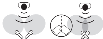
Обычные стерео-микрофоны
