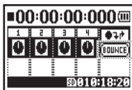
Иконка BOUNCE
