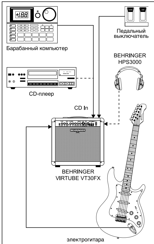
Рис. 3.1: Стандартный сетап с VT30FX
