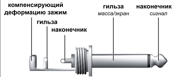
Рис. 4.1: 6,3-мм моноштекер
