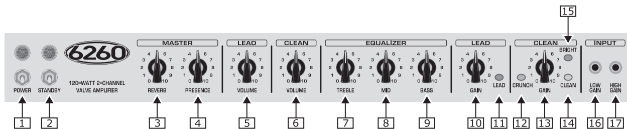
Передняя панель BUGERA 6260
